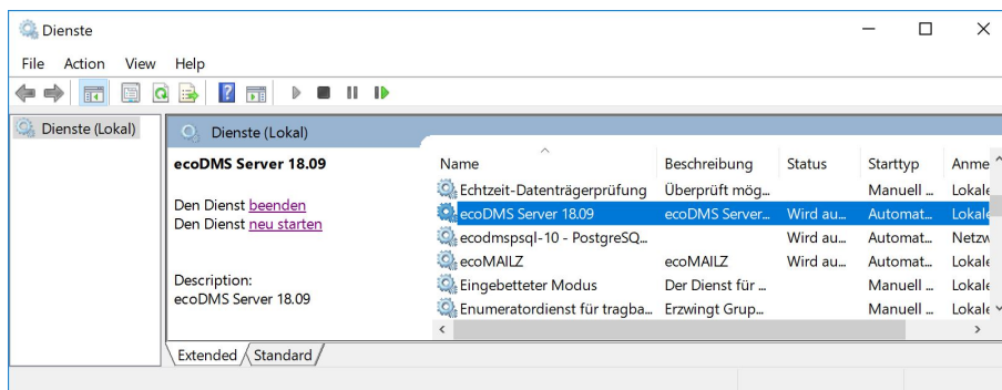
Abb. (ähnlich) 14.1: ecoDMS Server Dienst stoppen unter Windows
